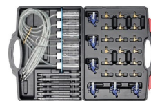
НАБОР ДИАГНОСТИЧЕСКИЙ К ФОРСУНКАМ COMMON RAIL
